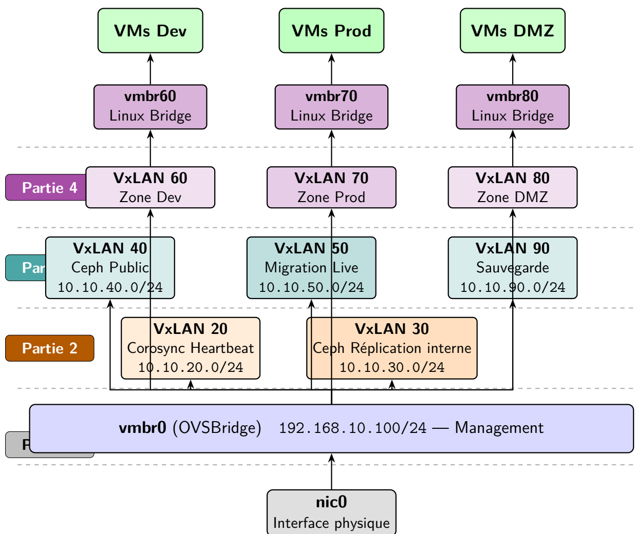
FIGURE IV.41 – Vue d'ensemble de la configuration réseau de PVE-01 — Quatre parties logiques
